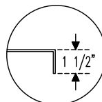
Flat Edge Both Sides
