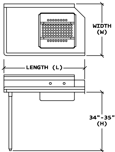
Left Side
