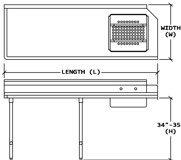
Left Side
